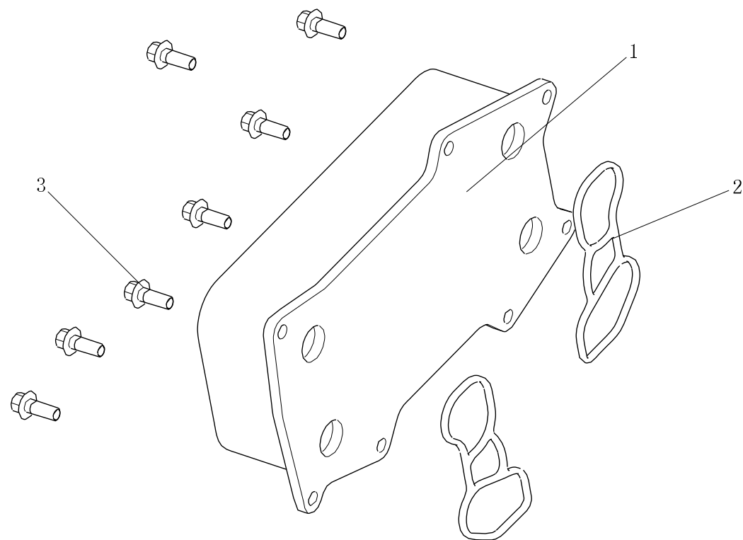
图 24 机油冷却器逻辑总成
