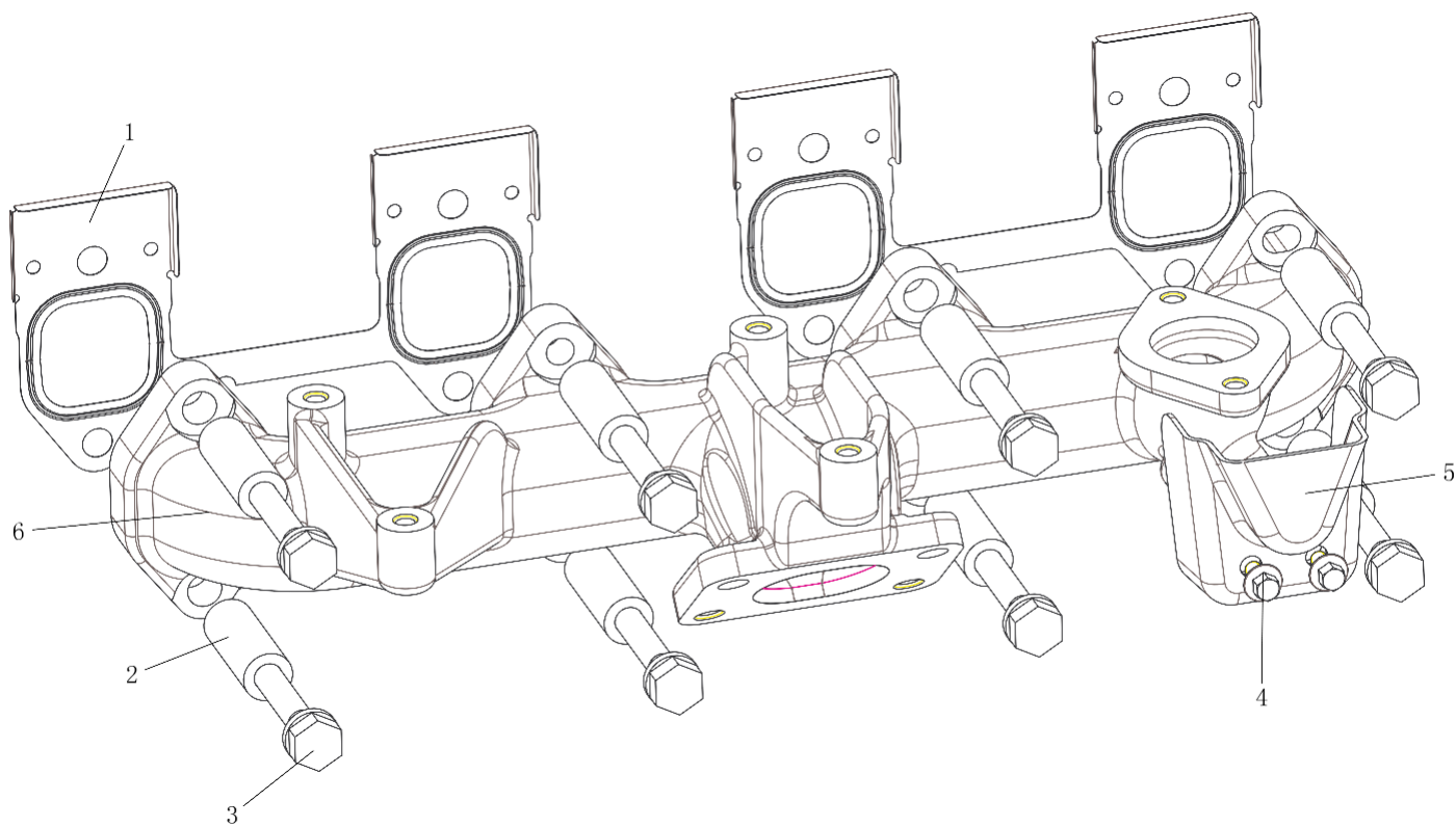
图 10 排气歧管逻辑总成
