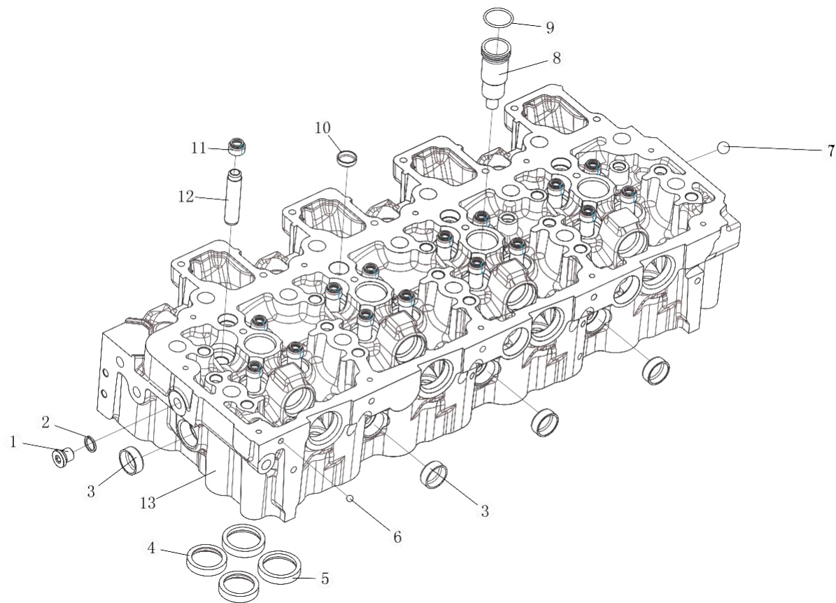
图 6 气缸盖分装总成
