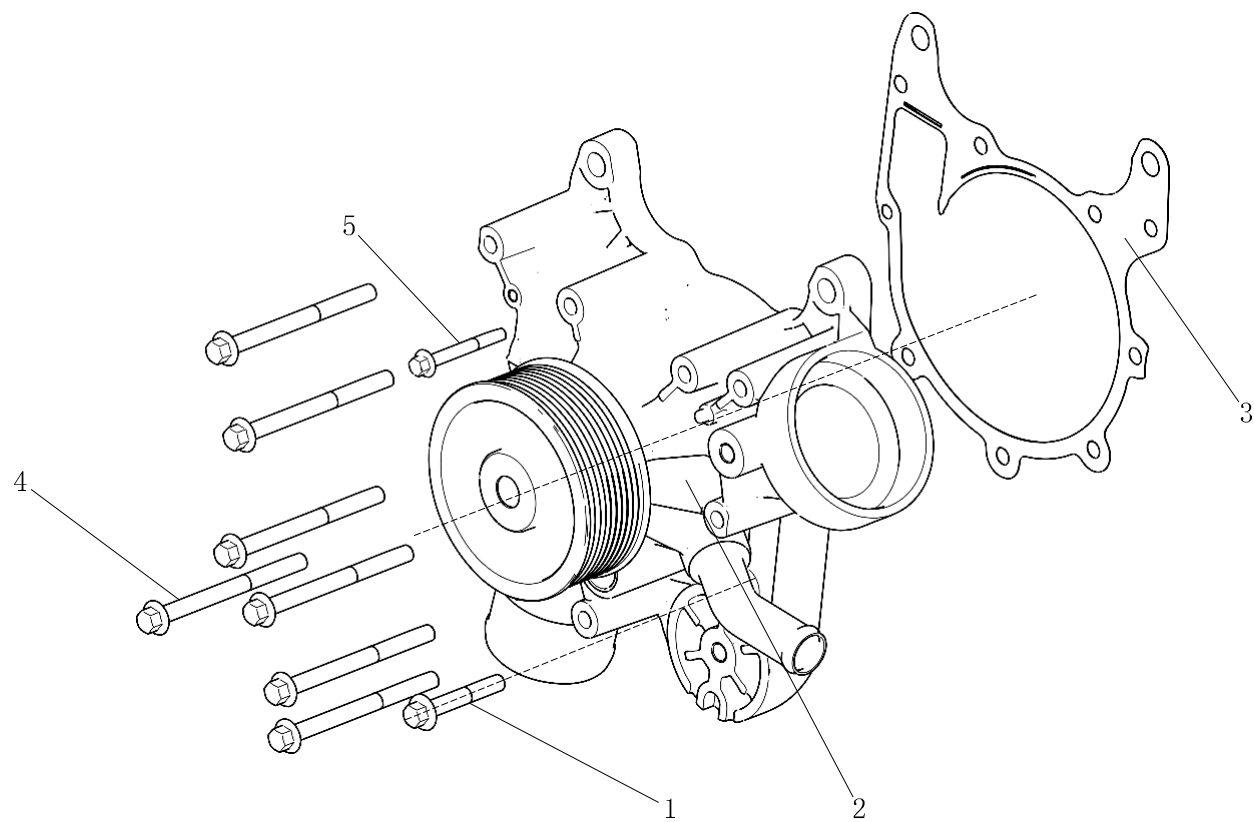
图 27 水泵逻辑总成
