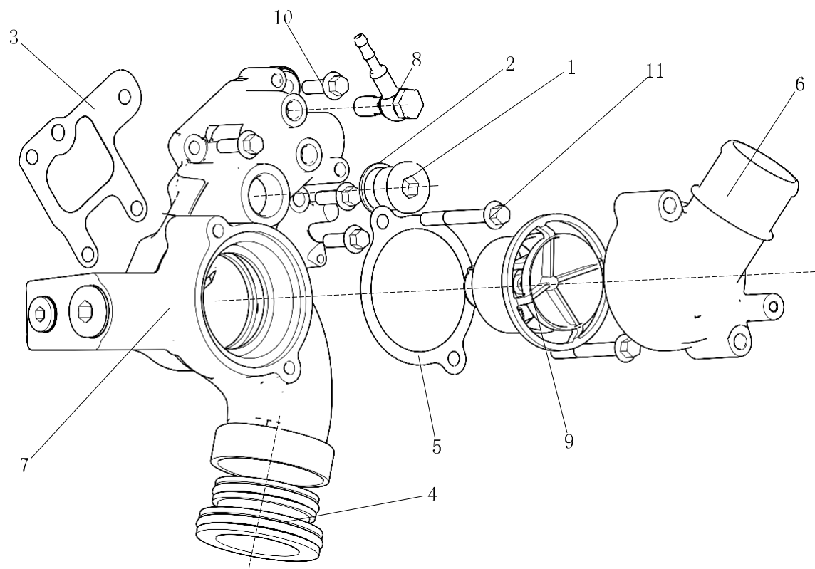
图 26 冷却系管路逻辑总成
