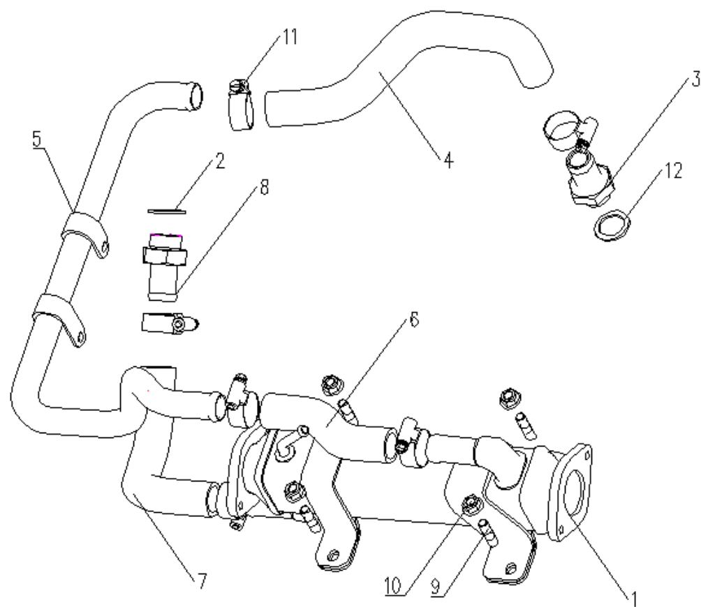
图 25 EGR 冷却器逻辑总成
