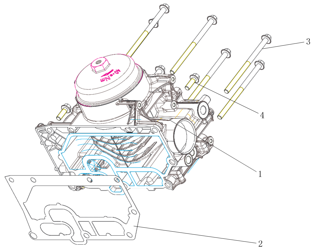
图 18 机油滤清器逻辑总成
