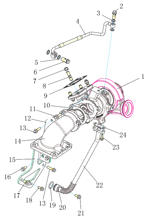
图 21 增压器
