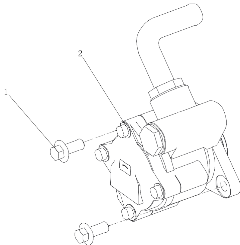
图 28 动力转向油泵逻辑总成
