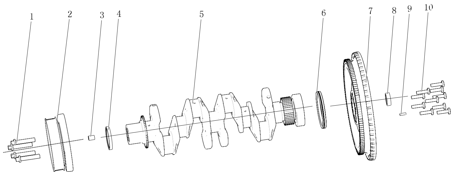
图 12 曲轴及飞轮组件
