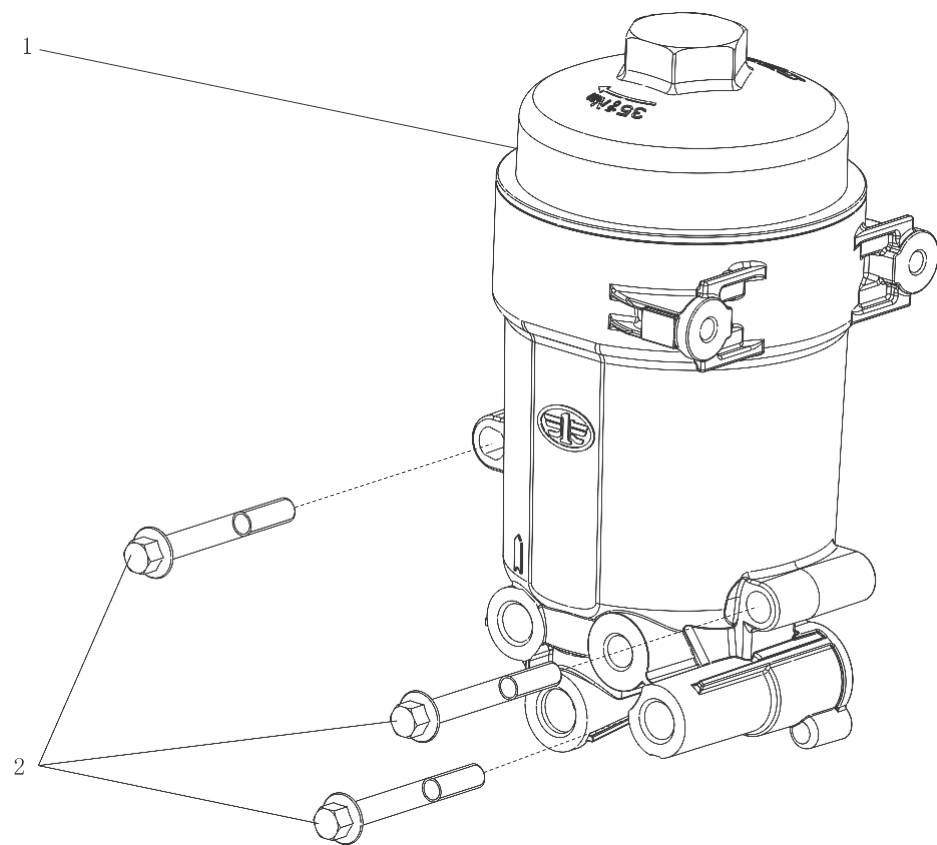
图 20 燃油细滤器
