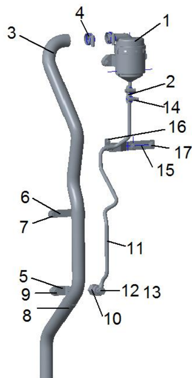
图 19 曲轴箱通风系统逻辑总成
