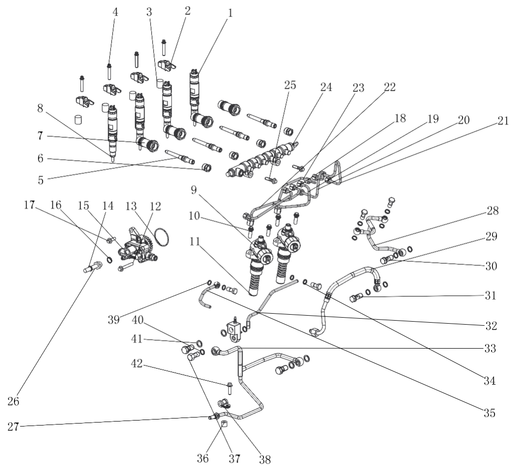
图 22 发动机供油系逻辑总成
