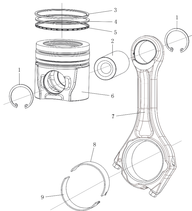
图 11 活塞连杆组件
