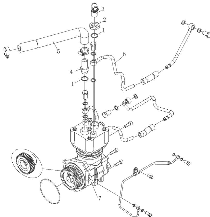
图 29 空气压缩机
