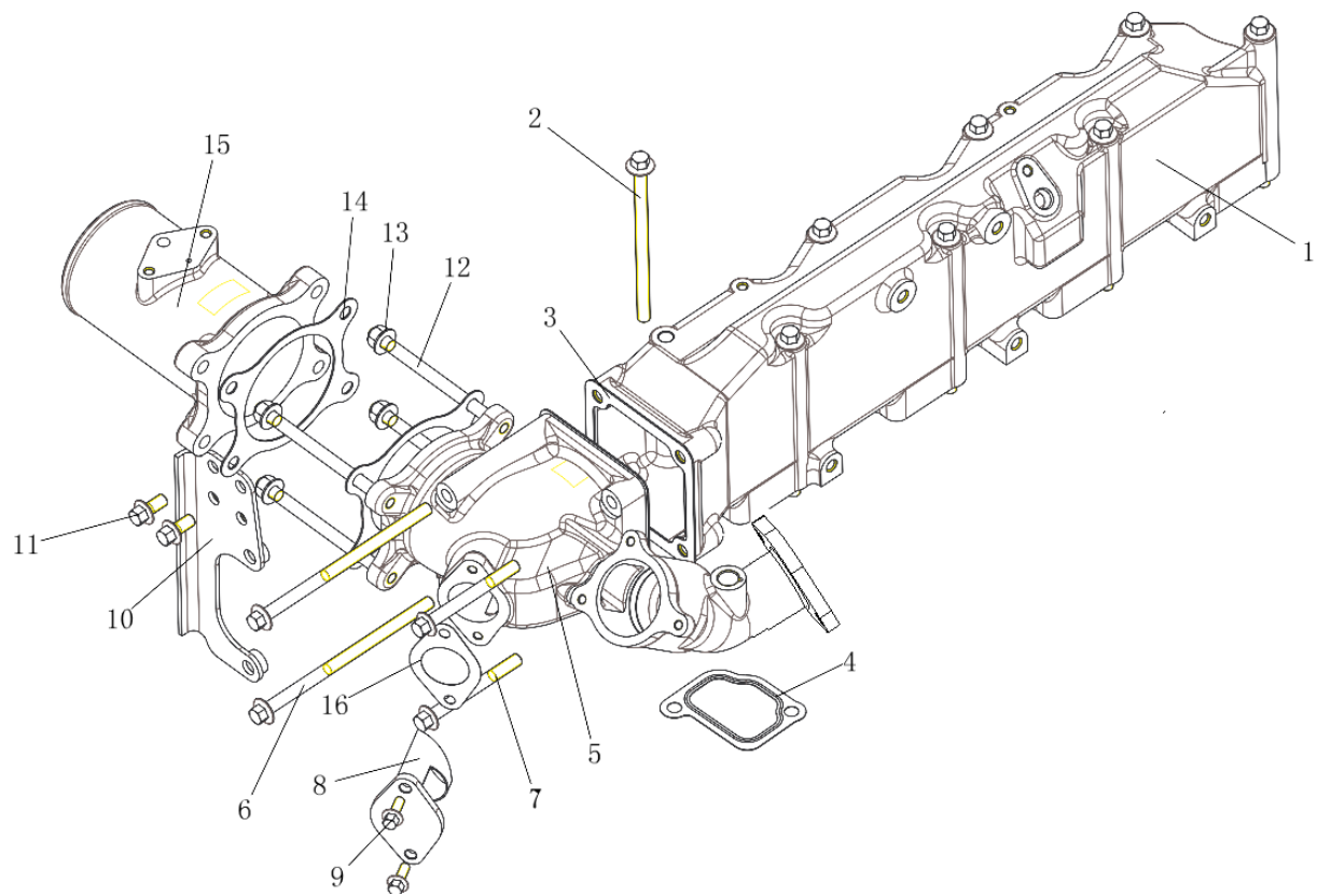
图 9 进气歧管逻辑总成
